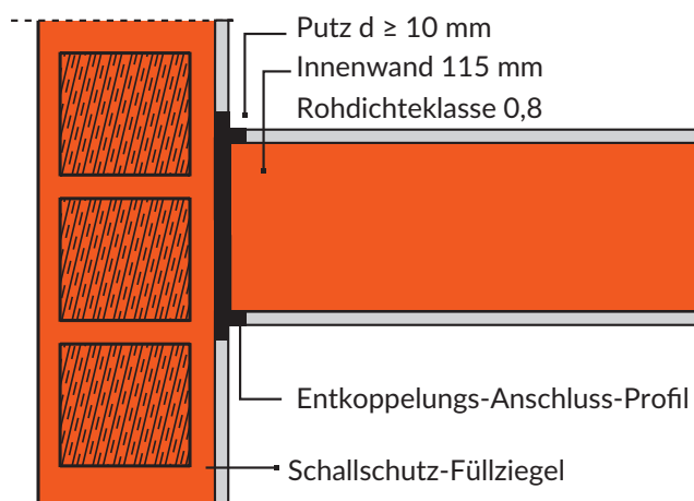
Bild 22: ZIS - Ziegel-Innenwand-System
