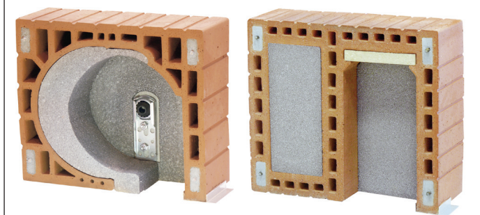
Bild 15: Ziegel-Rollladenkasten (Beispiele)
